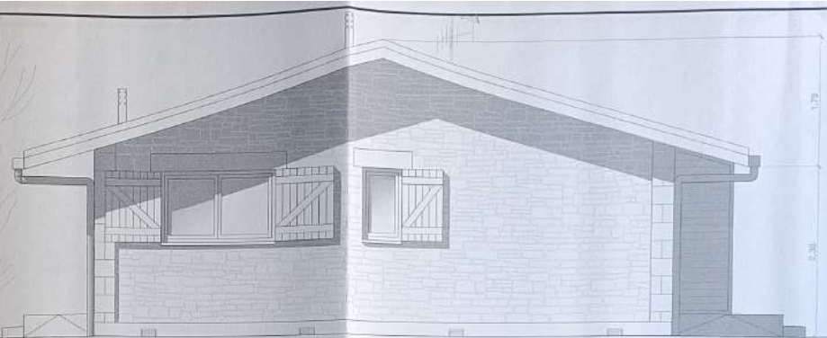
ALZADO SUROESTE
