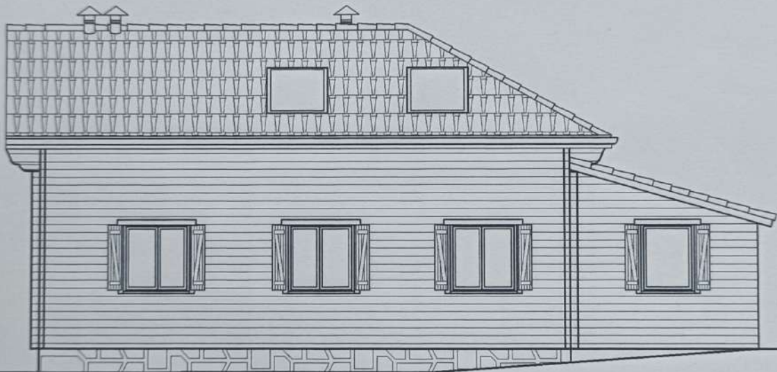
ALZADO POSTERIOR
