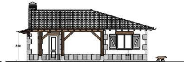
ALZADO ESTE
