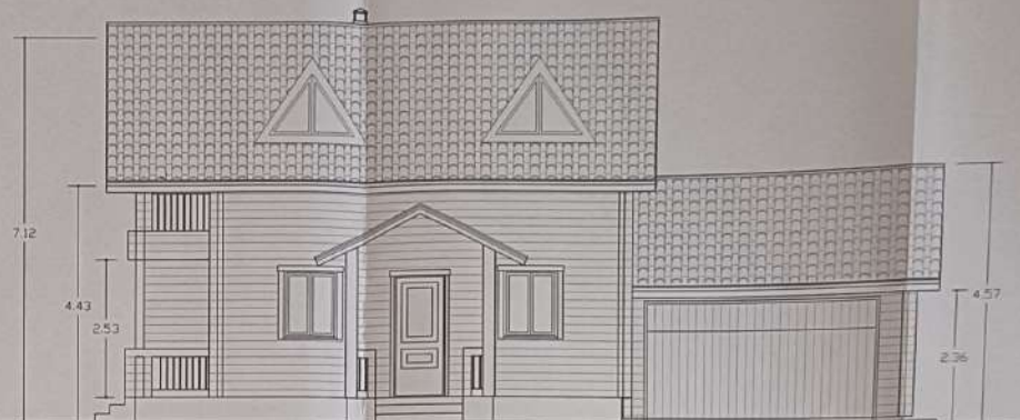
ALZADO SUR
