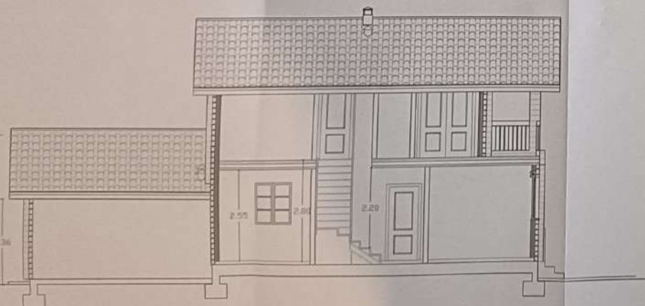
SECCION -AA-
