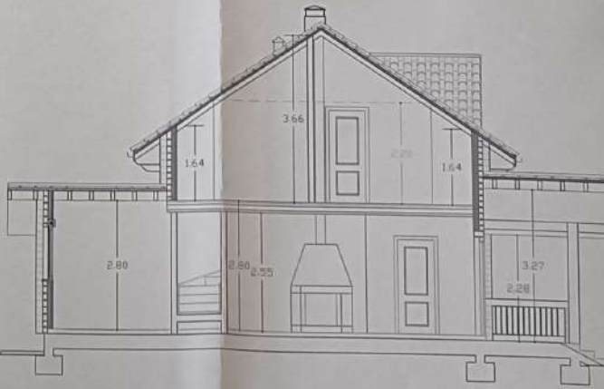
SECCION -BB-
