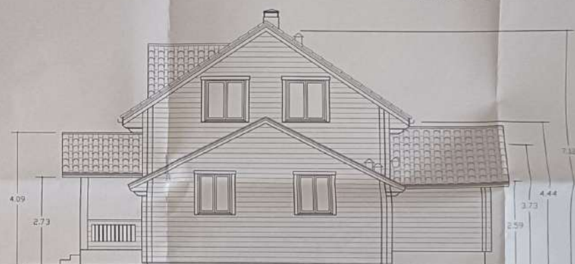
ALZADO OESTE
