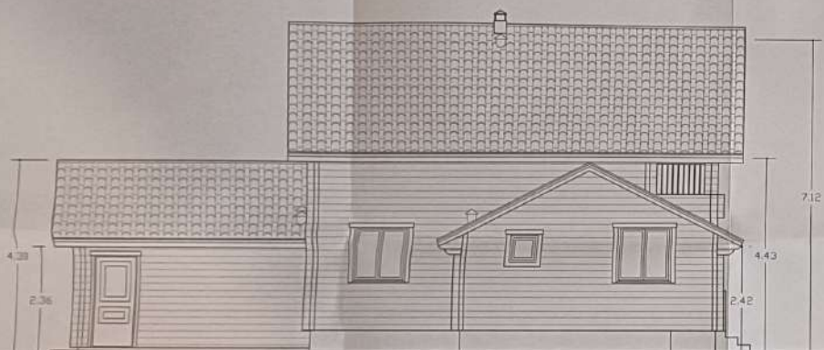
ALZADO NORTE
