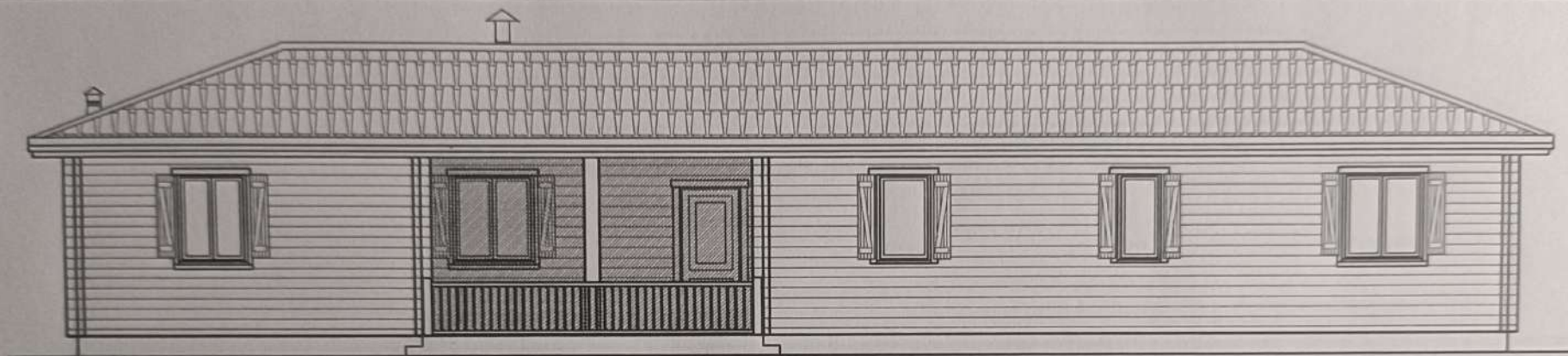
ALZADO FRONTAL
