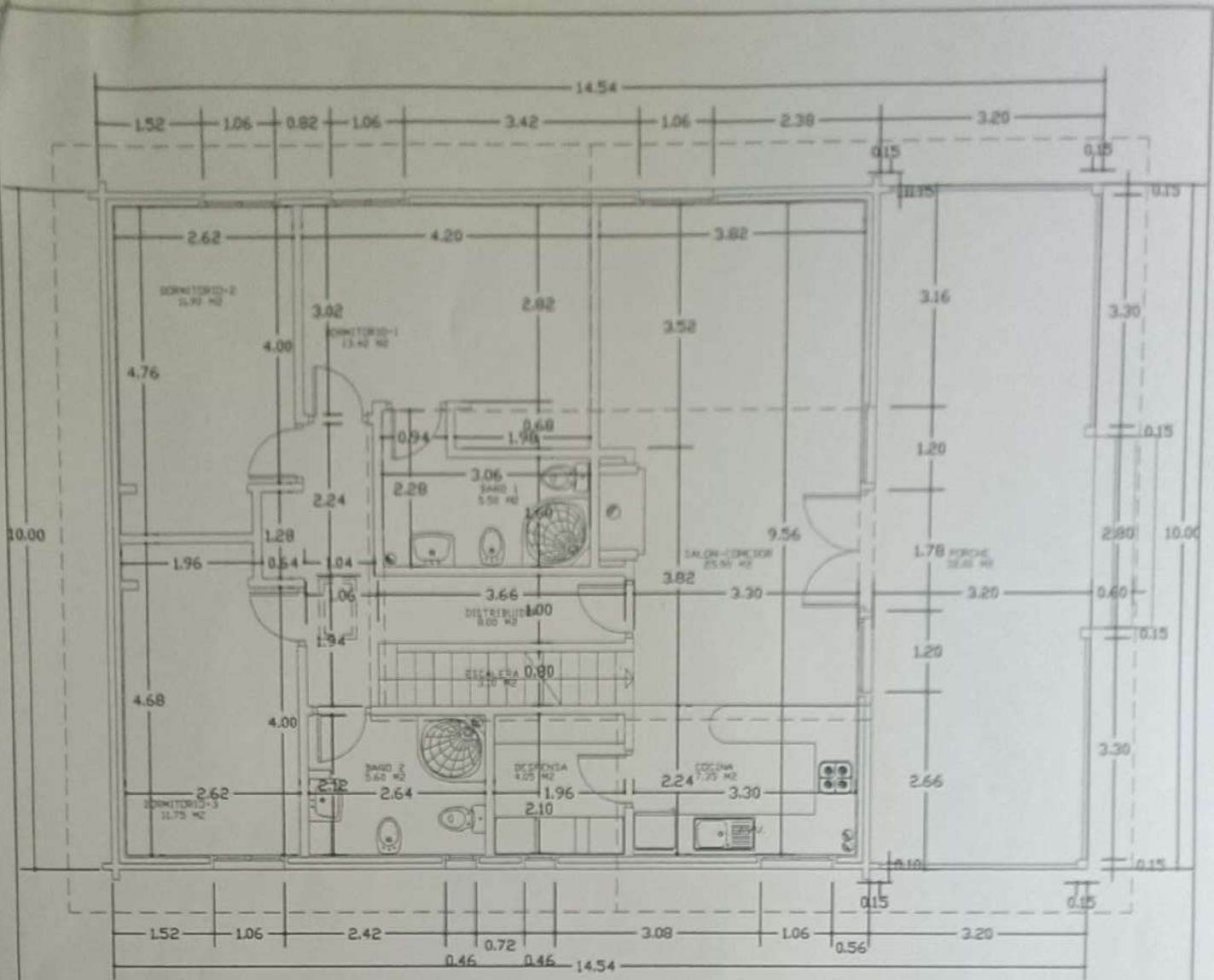
PLANTA BAJA
