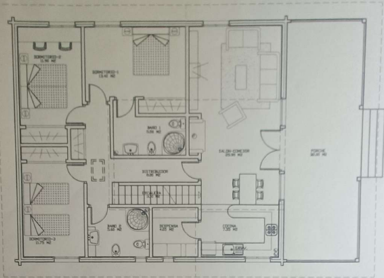
PLANTA BAJA
