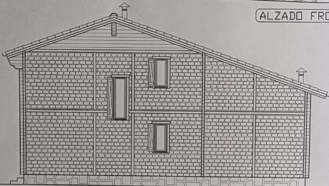
ALZADO POSTERIOR
