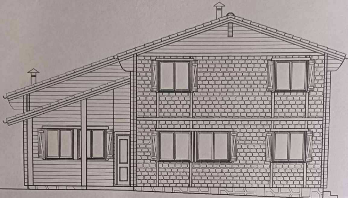
ALZADO FRONTAL
