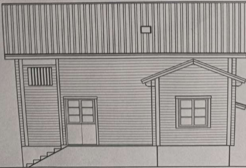
ALZADO LATERAL
