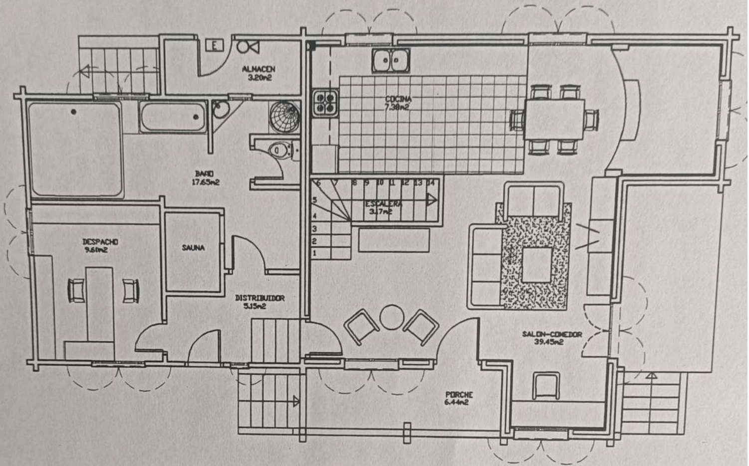
PLANTA BAJA
