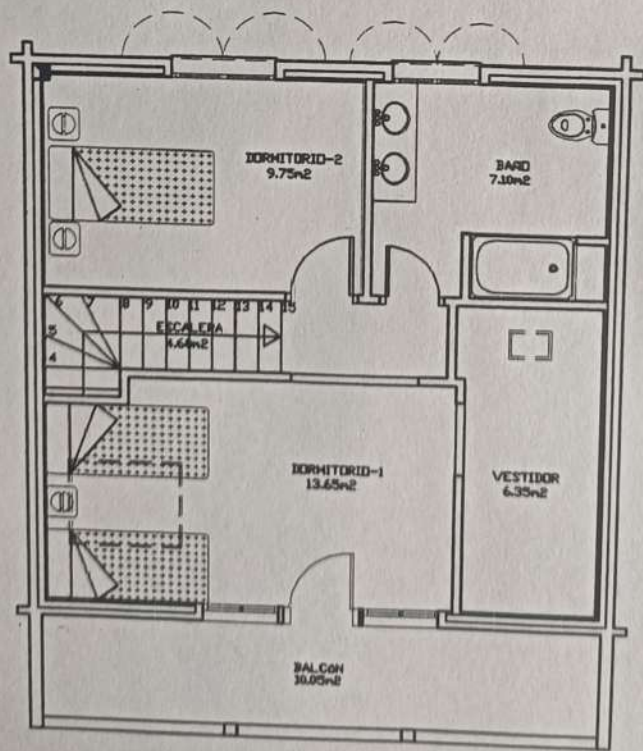
PLANTA PRIMERA
