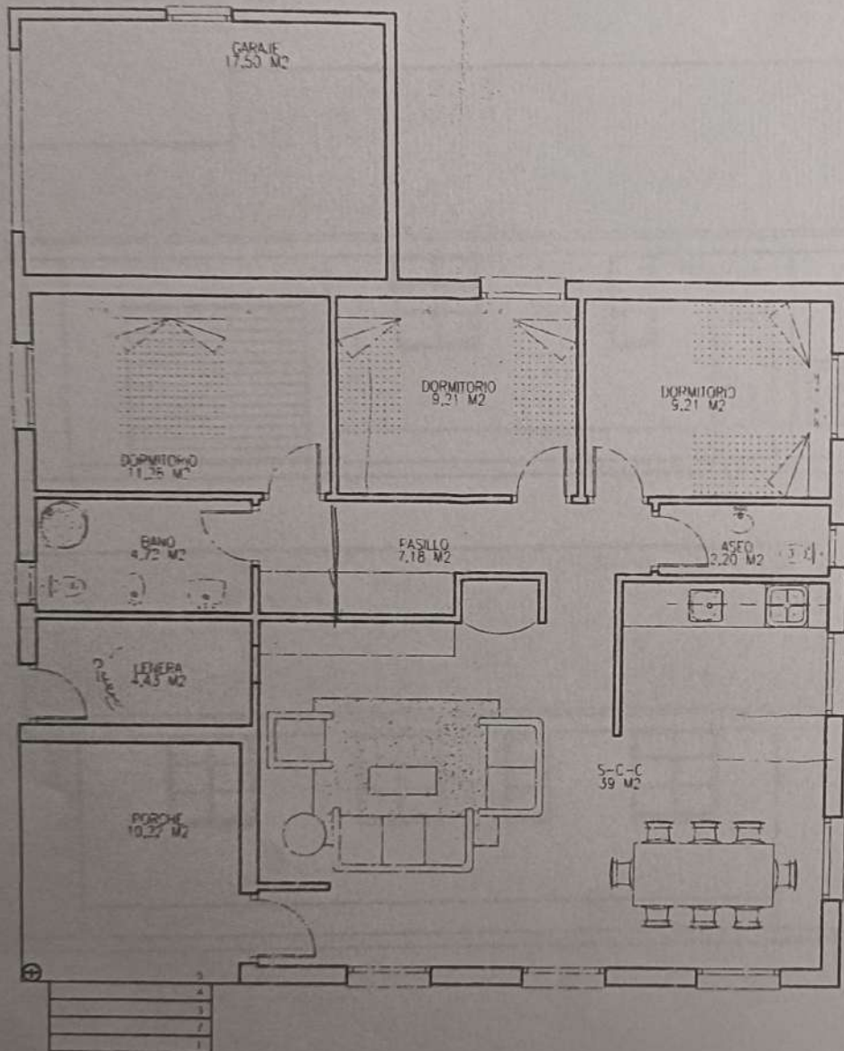
PLANTA BAJA
