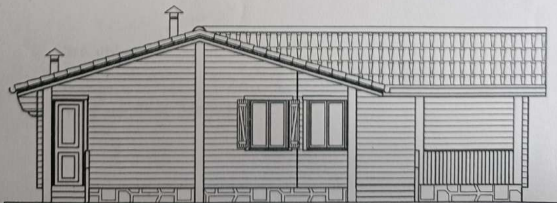
ALZADO LATERAL
