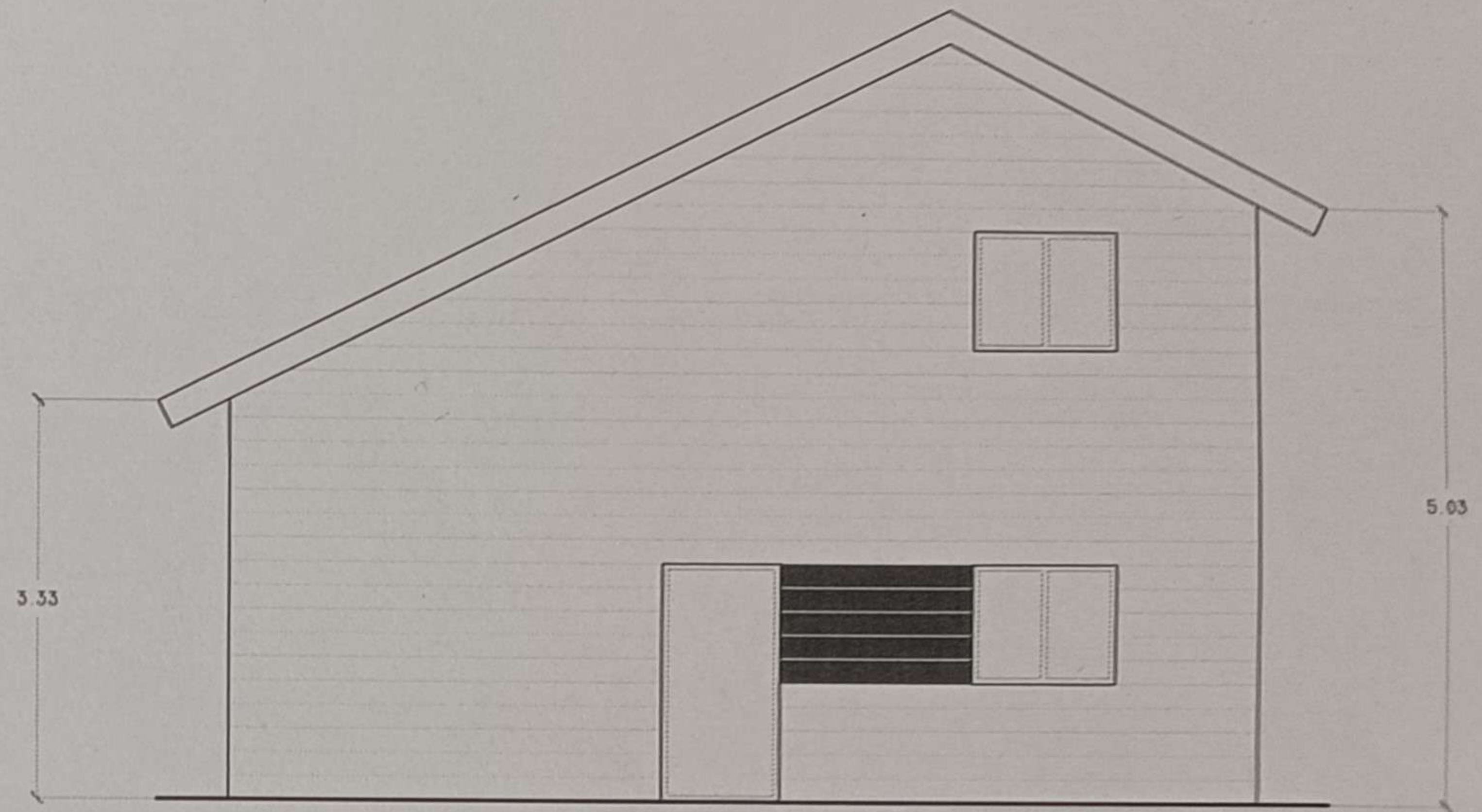
ALZADO ESTE
