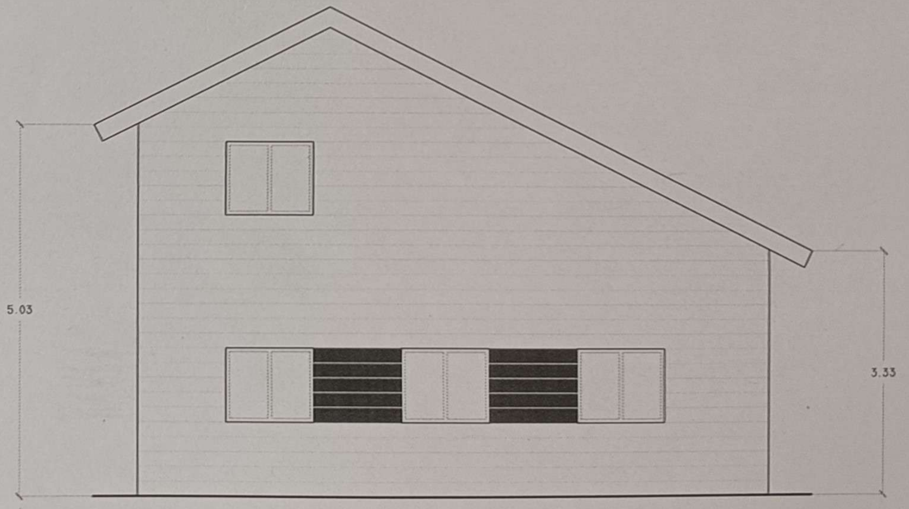
ALZADO OESTE
